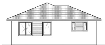
ZÁPADNÝ POHĽAD
